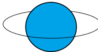
Neptun
