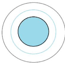
Uranus & seine runden Monde
