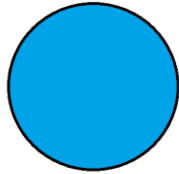
Erde
